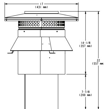
CT-3A-B
