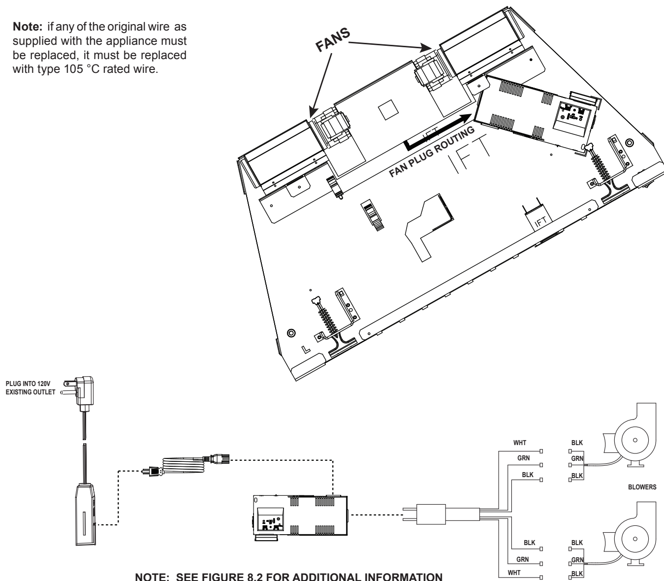
Figure 8.3 Fan Wiring Diagram
