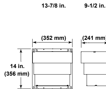
DRC-RADIUS Cap Shield
