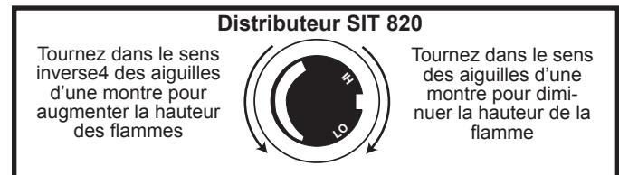
Fig. 55 Bouton de réglage des flammes pour le distributeur SIT.
