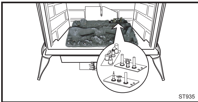
Fig. 54 emplacement de la veilleuse.
