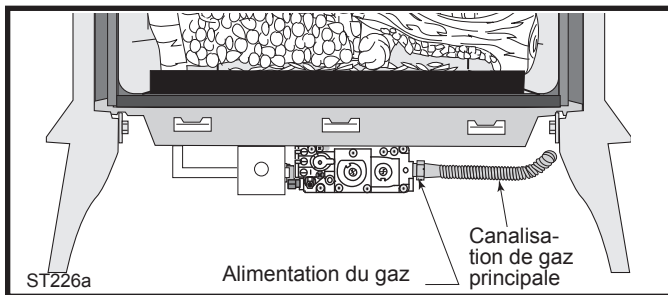
Fig. 69 Raccordez la canalisation de gaz au côté gauche du distributeur.
