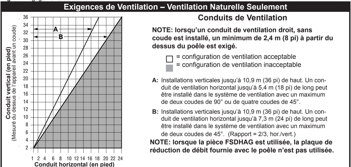
12 Fig. 11 Sortie du conduit de ventilation – ventilation naturelle SEULEMENT.
