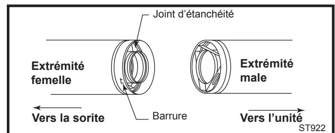
Fig. 33 Joint de connexion.
