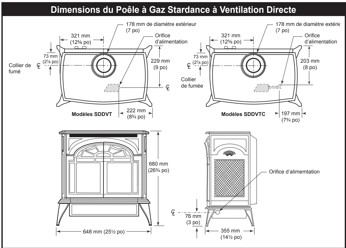
Fig. 1 Dimensions du poêle Stardance.
