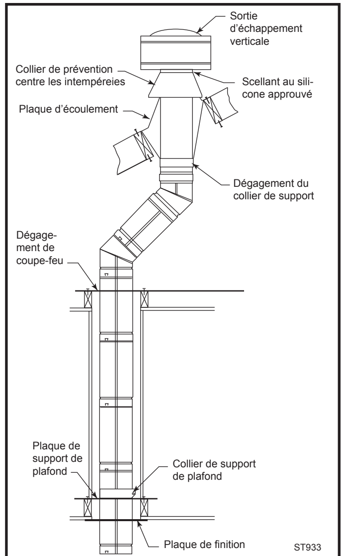
Fig. 43 Configuration typique de ventilation verticale.
