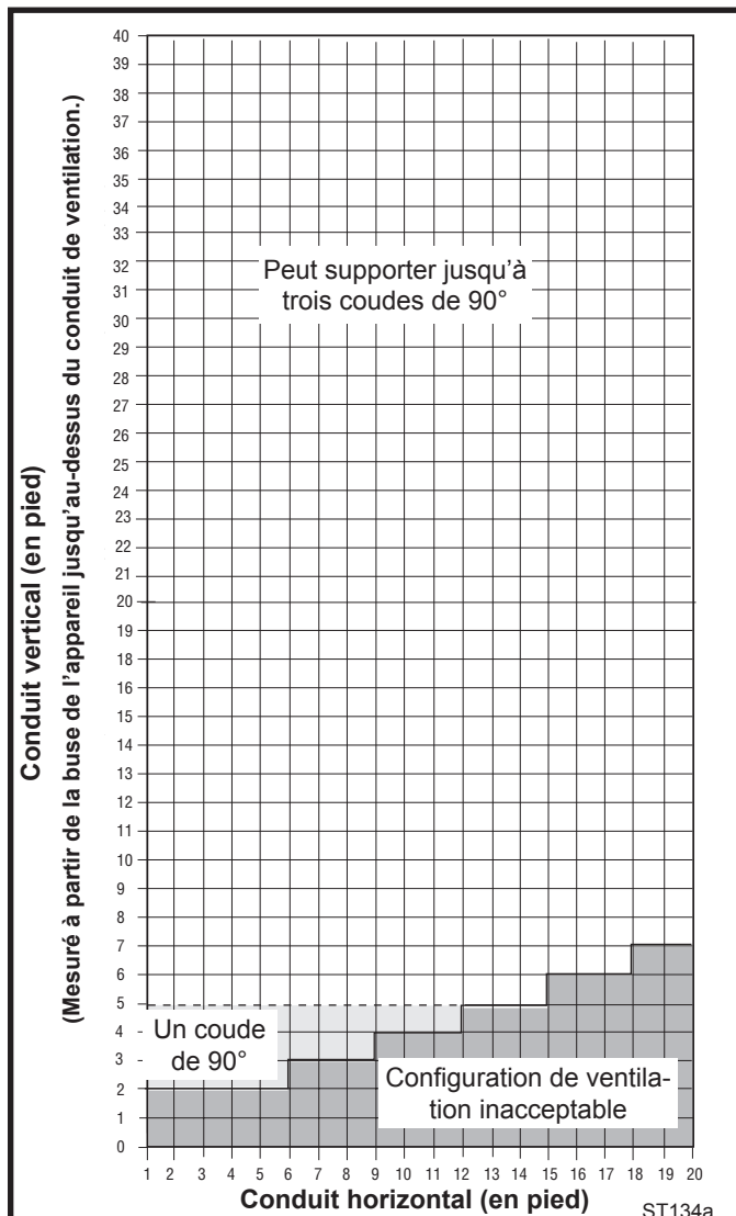
Fig. 7 Sortie du conduit de ventilation horizontal.
