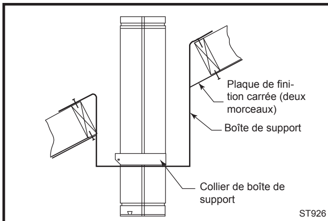
Fig. 36 Boîte de support.
