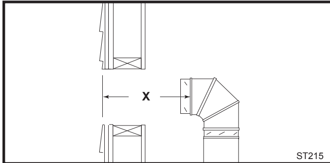
Fig. 26 Mesurez la longueur horizontale.
