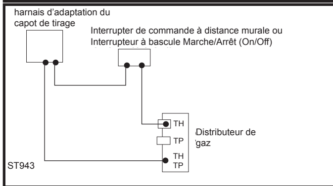
Fig. 88 Câblage de l'adaptateur du capot de tirage.
