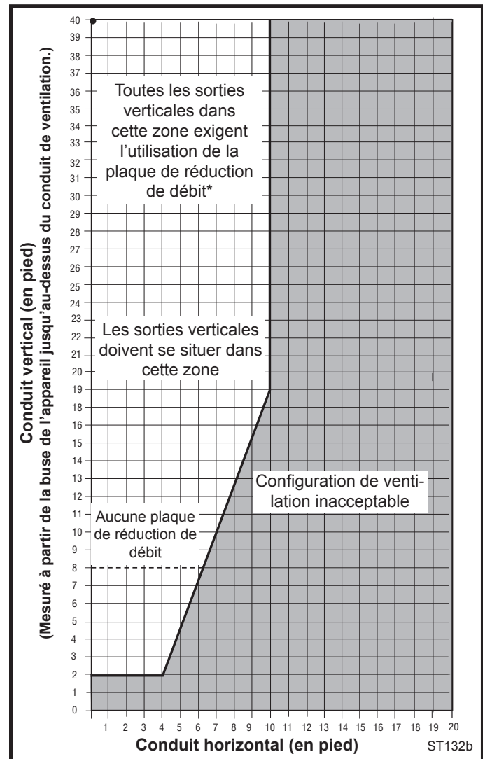
Fig. 8 Sortie du ventilation vertical.
