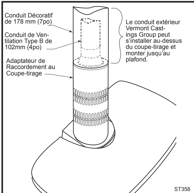
Fig. 45 Conduit décoratif de 178mm (7po) enveloppant le conduit de ventilation type B.
