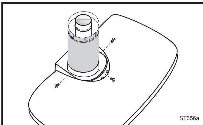
Fig. 22 Installation du conduit de raccordement extérieur DuraVent.
