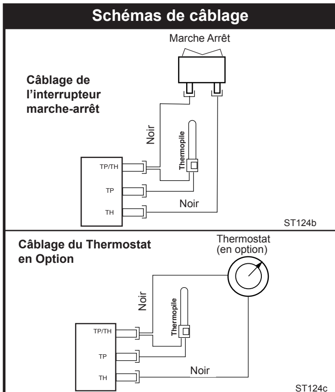
Fig. 87 Interrupteur marche-arrêt et circuit du thermostat en option.
