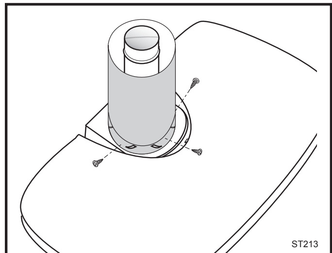
Fig. 20 Fixez le conduit extérieur au moyen des vis à tôle n° 12 x 1/2 po.
