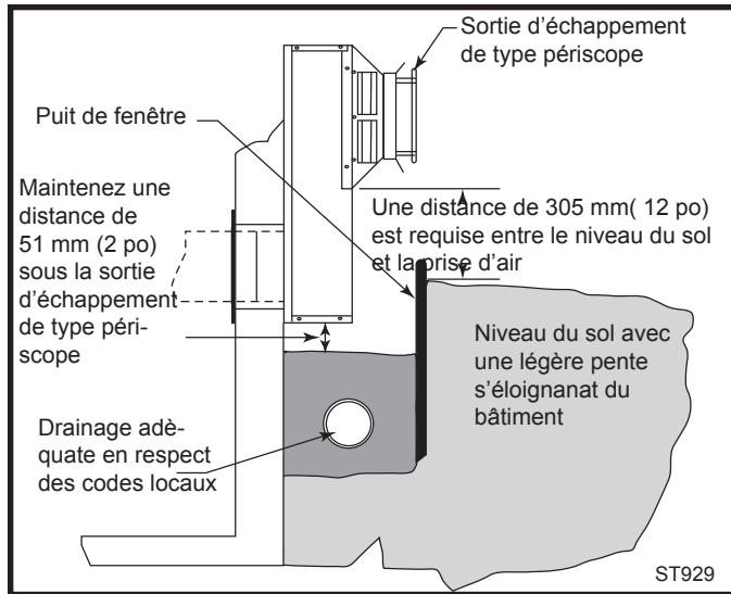
Fig. 39 Installation sous le niveau du sol.
