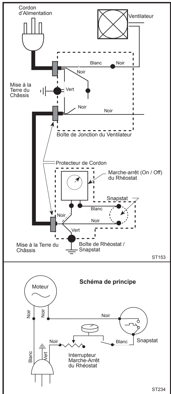
Fig. 89 Circuit du ventilateur Stardance.
