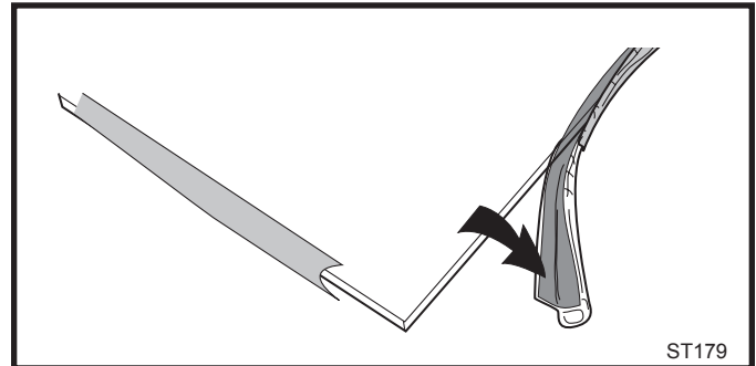
Fig. 85 Enveloppez le matériau d'étanchéité autour du rebord extérieur du panneau vitré.
