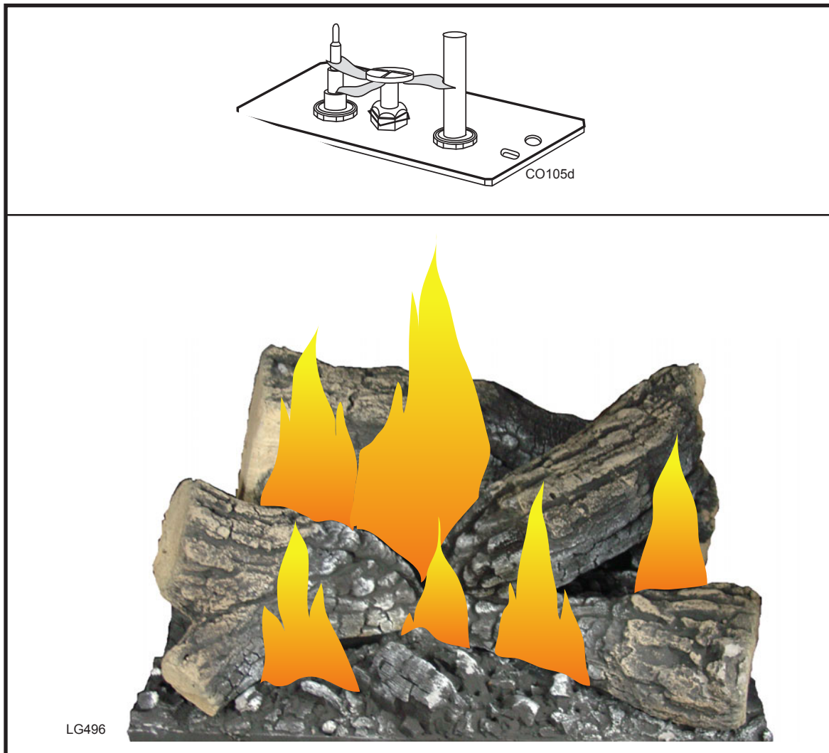
Fig. 56 Forme idéale des flammes de la veilleuse et du brûleur.
