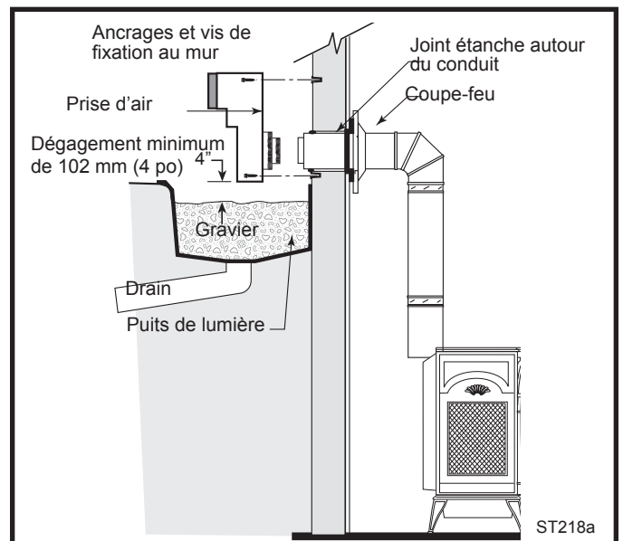
Fig. 29 Installation du nécessaire de prise d'air.
